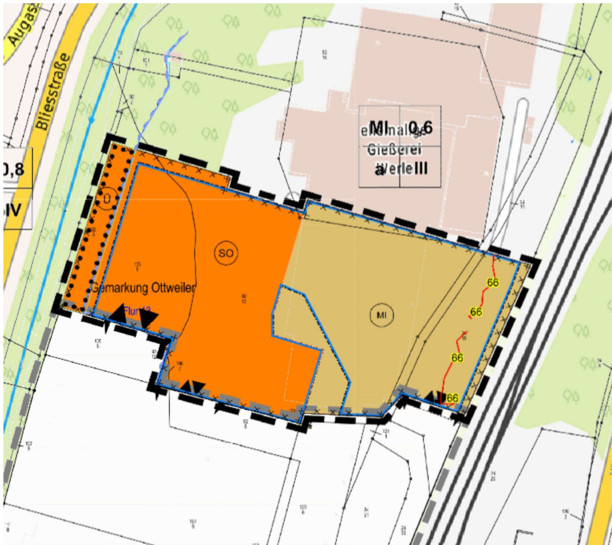
Bild 13c Maßgebliche Außenlärmpegel für sonstige Nutzung Berechnungshöhe 5,6 m (1. OG) Maßstab 1:1.500
