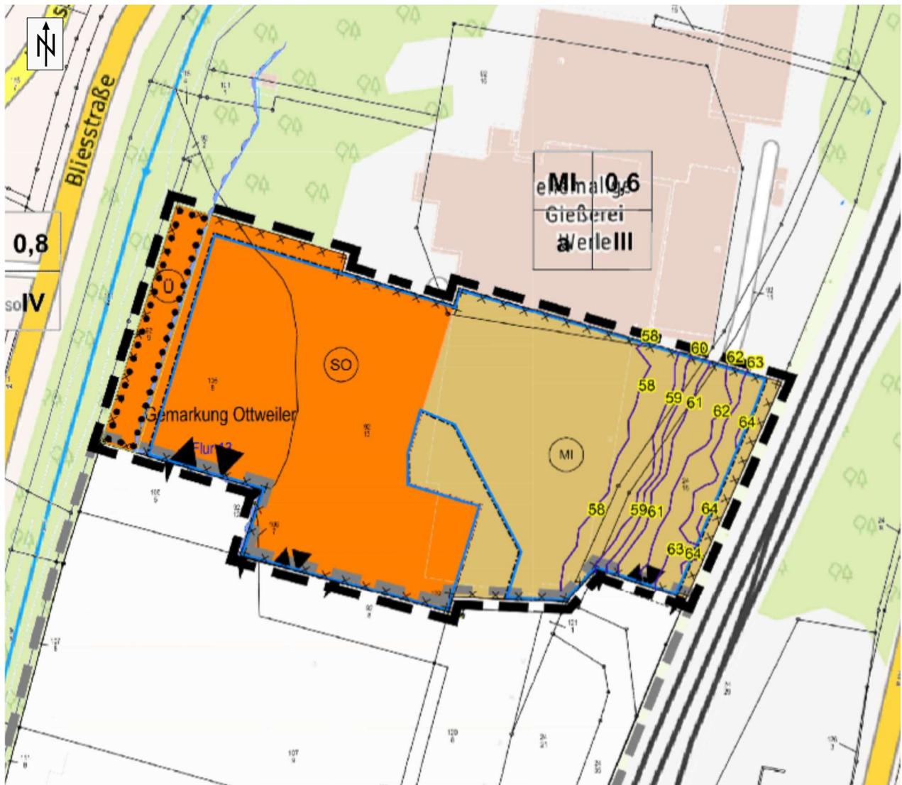
Bild 12a Beurteilungspegel Verkehrslärmimmissionen tags im Plangebiet (MI) Berechnungshöhe 5,6 m (1. OG) Maßstab 1:1.500
