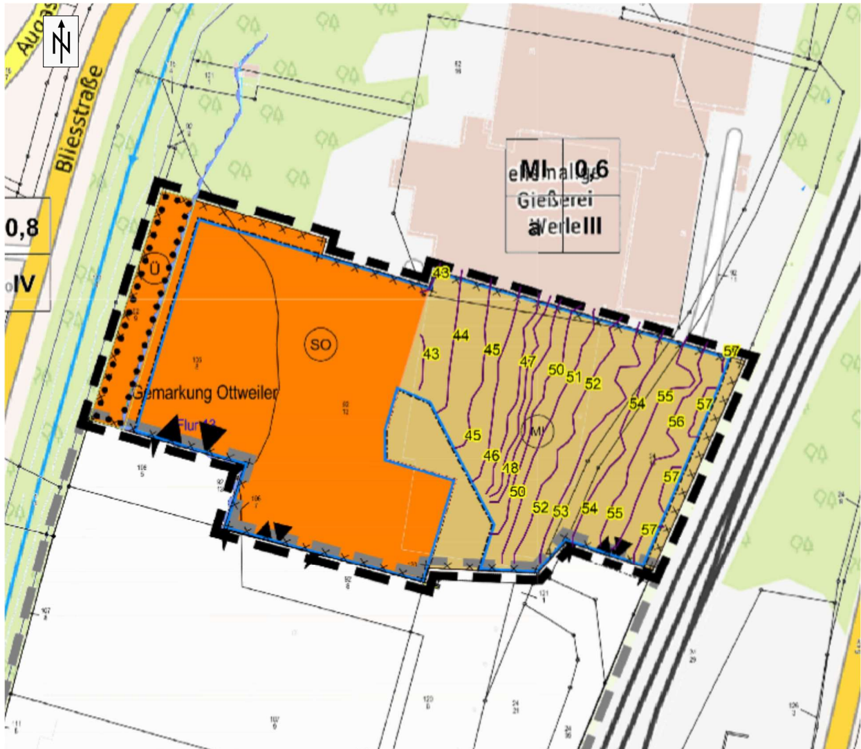
Bild 10d Beurteilungspegel Schienenverkehr nachts im Plangebiet (MI) Berechnungshöhe 11,2 m (3. OG) Maßstab 1:1.500
