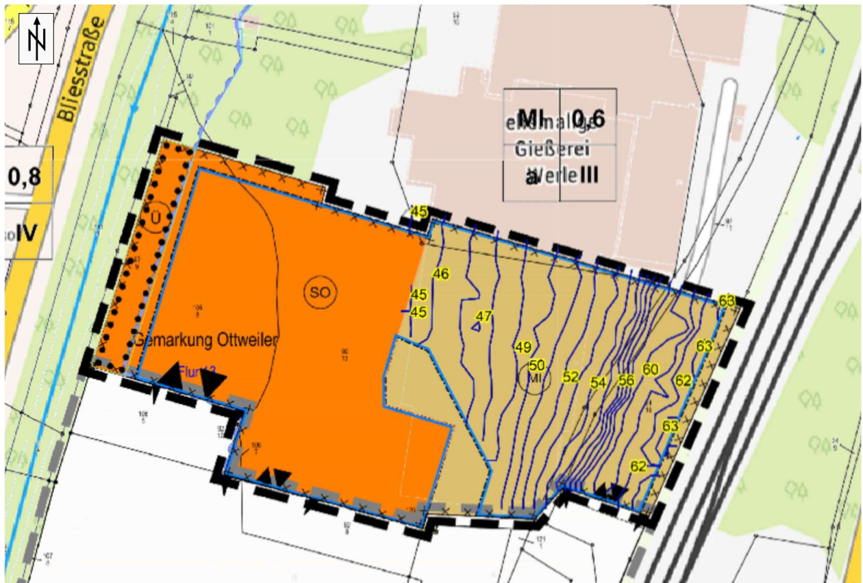
Bild 10a Beurteilungspegel Schienenverkehr tags im Plangebiet (MI) Berechnungshöhe 5,6 m (1. OG) Maßstab 1:1.500
