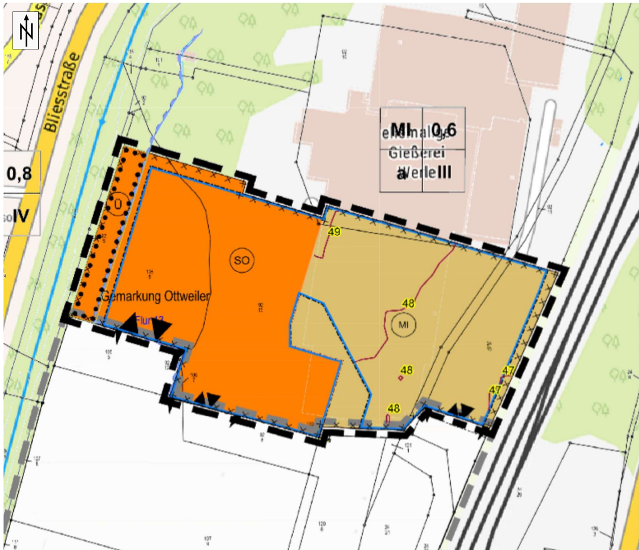
Bild 11c Beurteilungspegel Straßenverkehr nachts im Plangebiet (MI) Berechnungshöhe 5,6 m (1. OG) Maßstab 1:1.500
