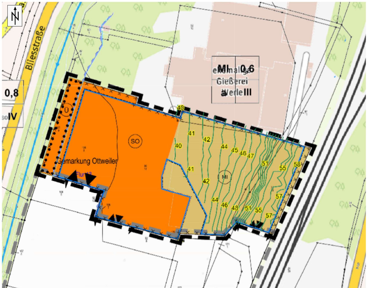
Bild 10c Beurteilungspegel Schienenverkehr nachts im Plangebiet (MI) Berechnungshöhe 5,6 m (1. OG) Maßstab 1:1.500
