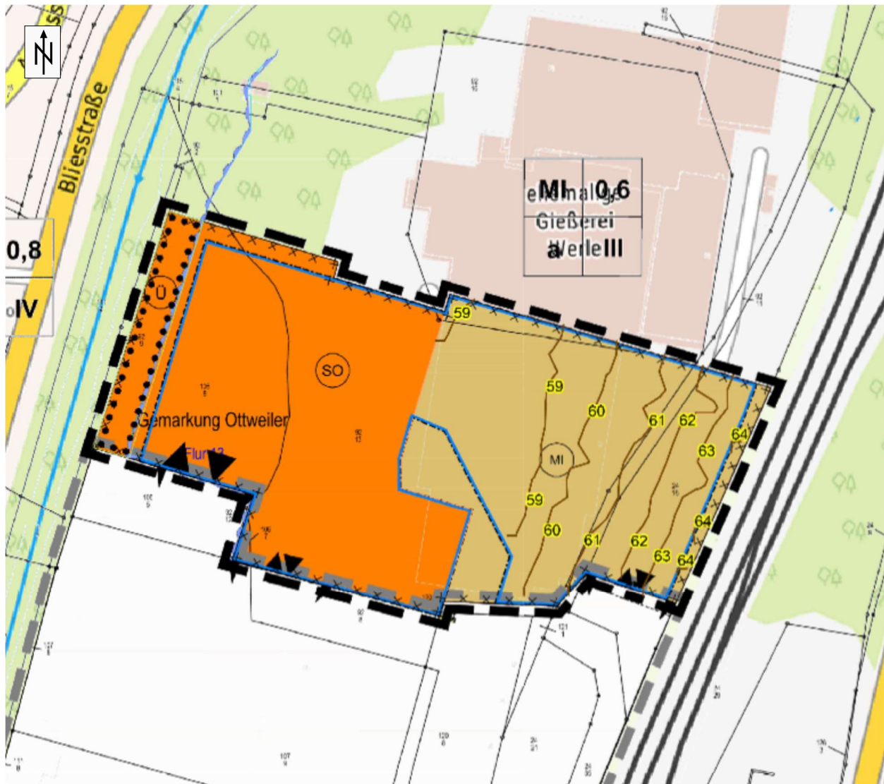
Bild 12b Beurteilungspegel Verkehrslärmimmissionen tags im Plangebiet (MI) Berechnungshöhe 11,2 m (3. OG) Maßstab 1:1.500
